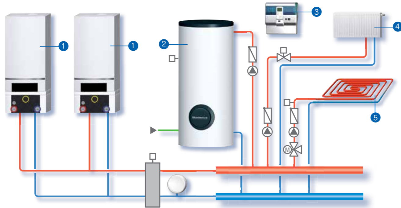
1 Logamax plus GB162 2 Boyler 3 Logamatic 4121 4 Radyatör 5 Yerden Isıtma
